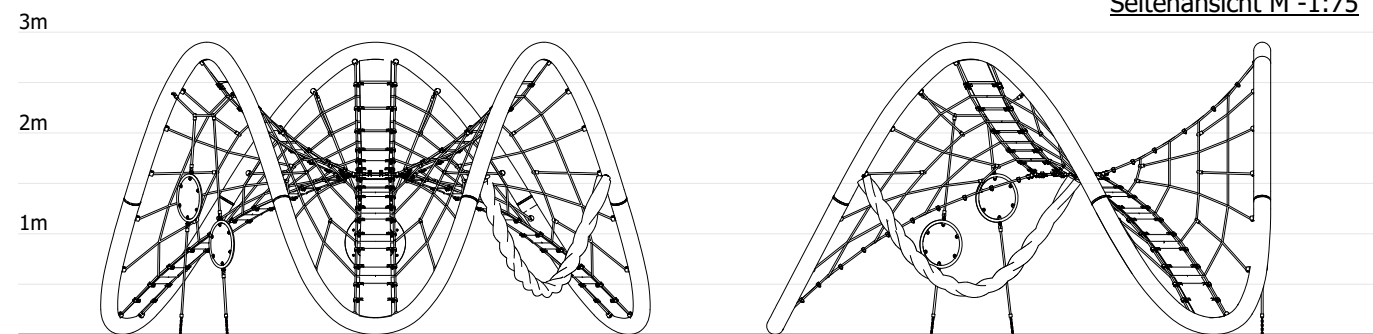
Seitenansicht M -1:75
