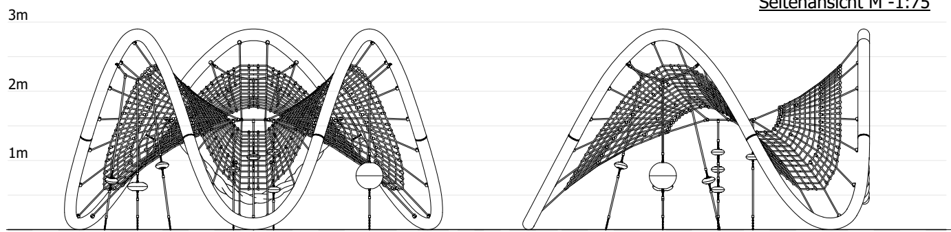
Seitenansicht M -1:75
