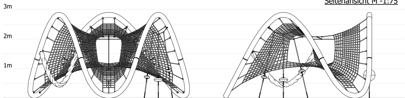
Seitenansicht M -1:75
