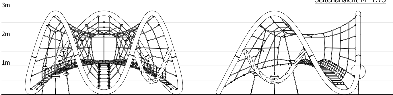
Seitenansicht M -1:75
