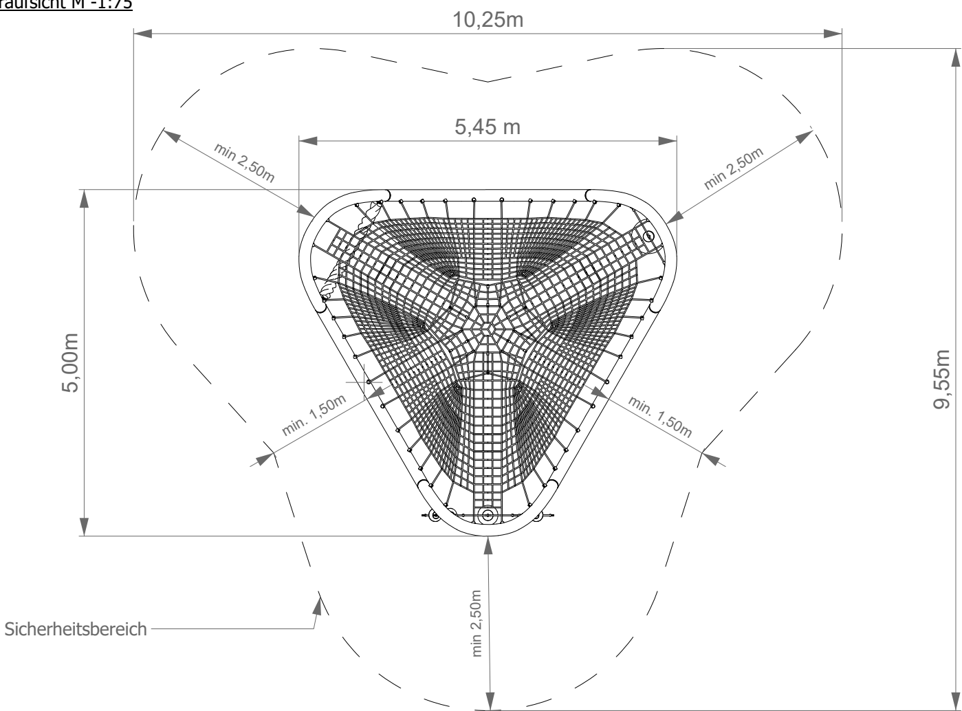
Draufsicht M -1:75
