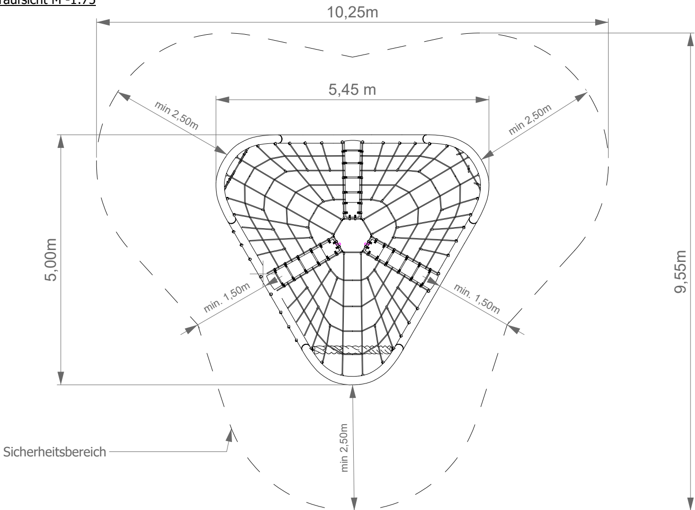
Draufsicht M -1:75
