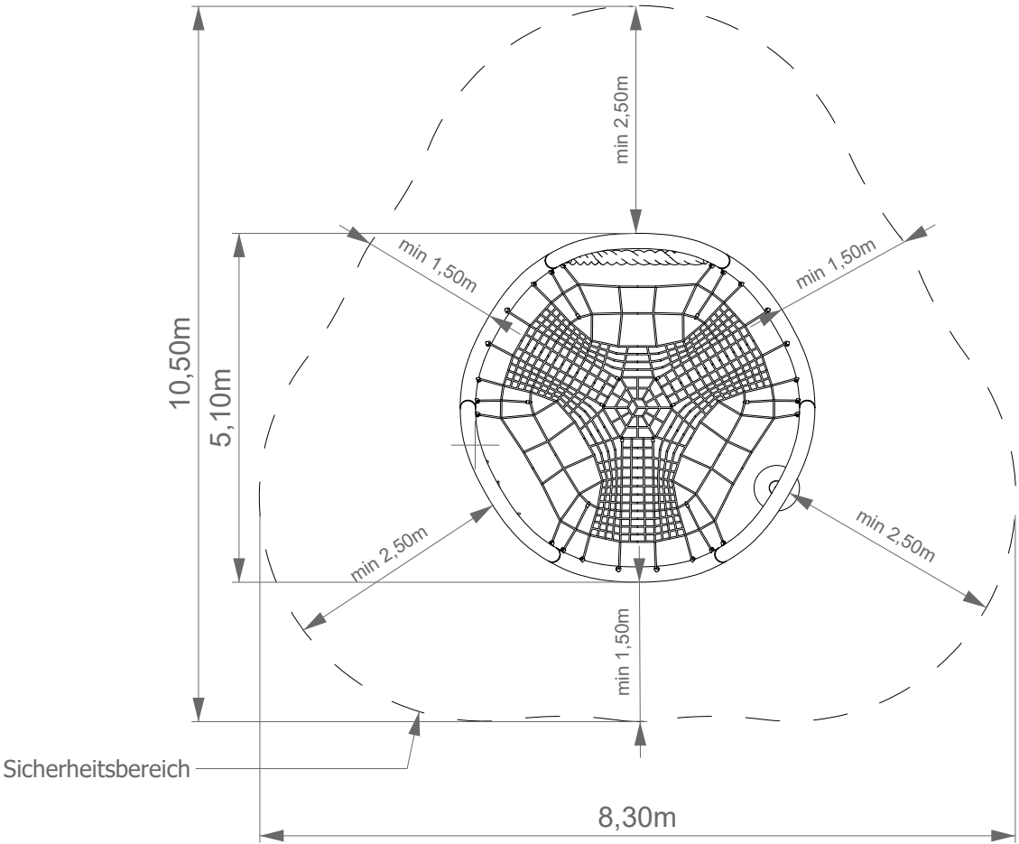
Draufsicht M -1:75
