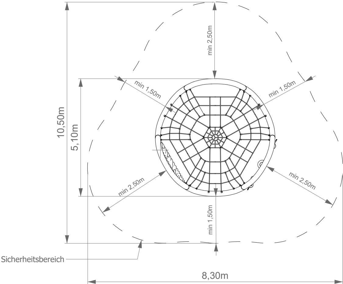
Draufsicht M -1:75
