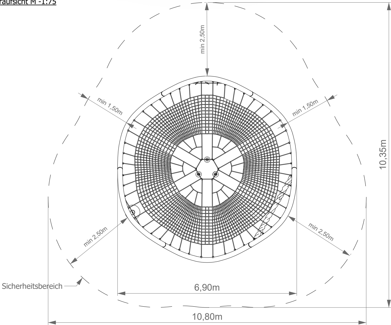
Draufsicht M -1:75
