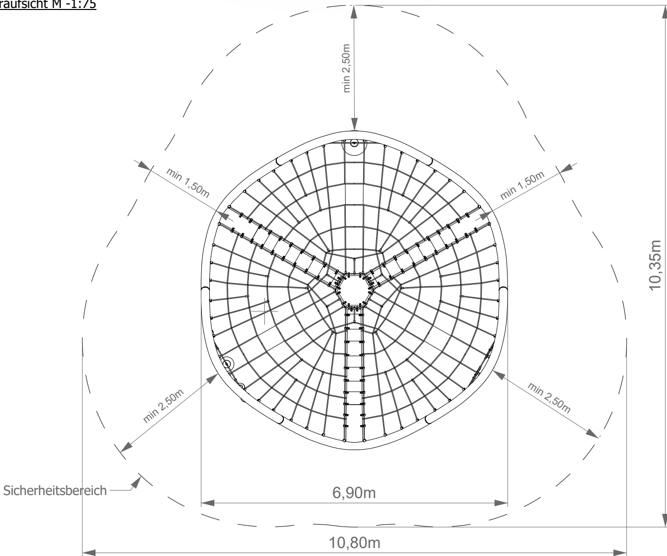
Draufsicht M -1:75
