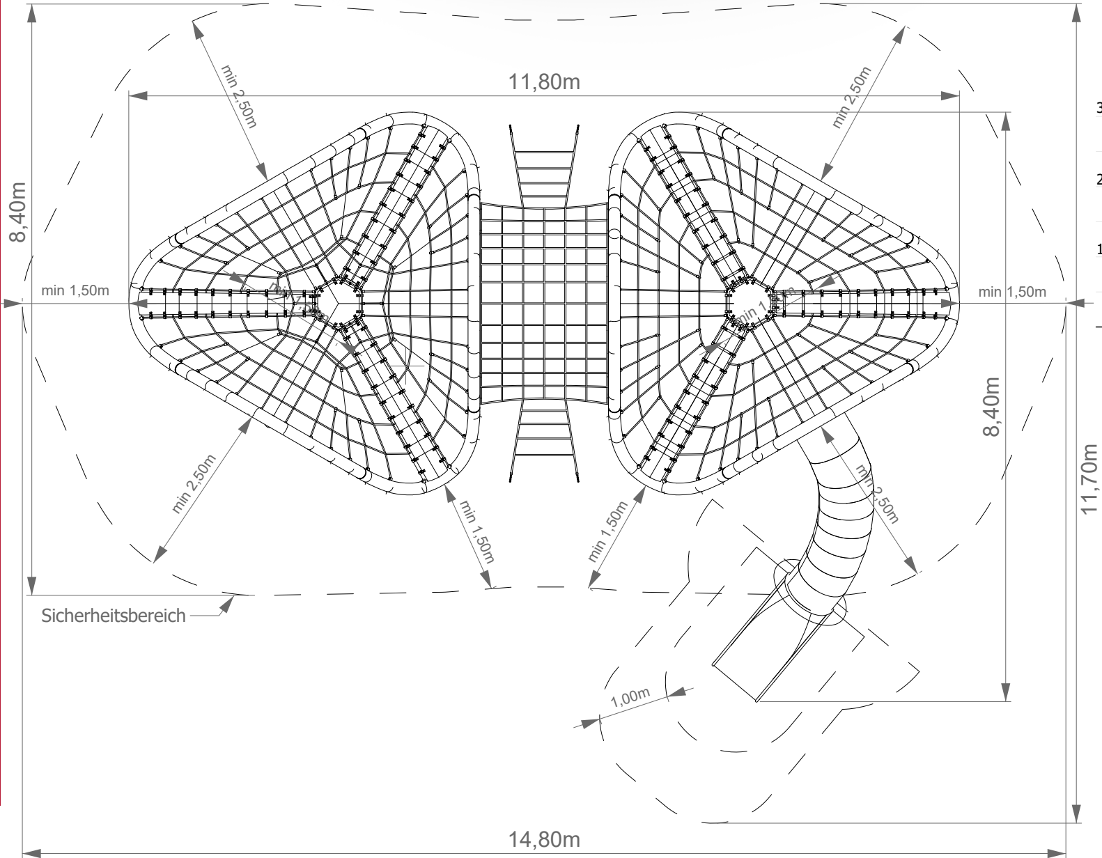
Draufsicht M -1:75
