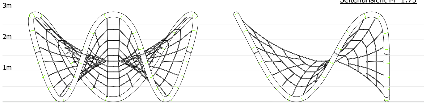
Seitenansicht M -1:75
