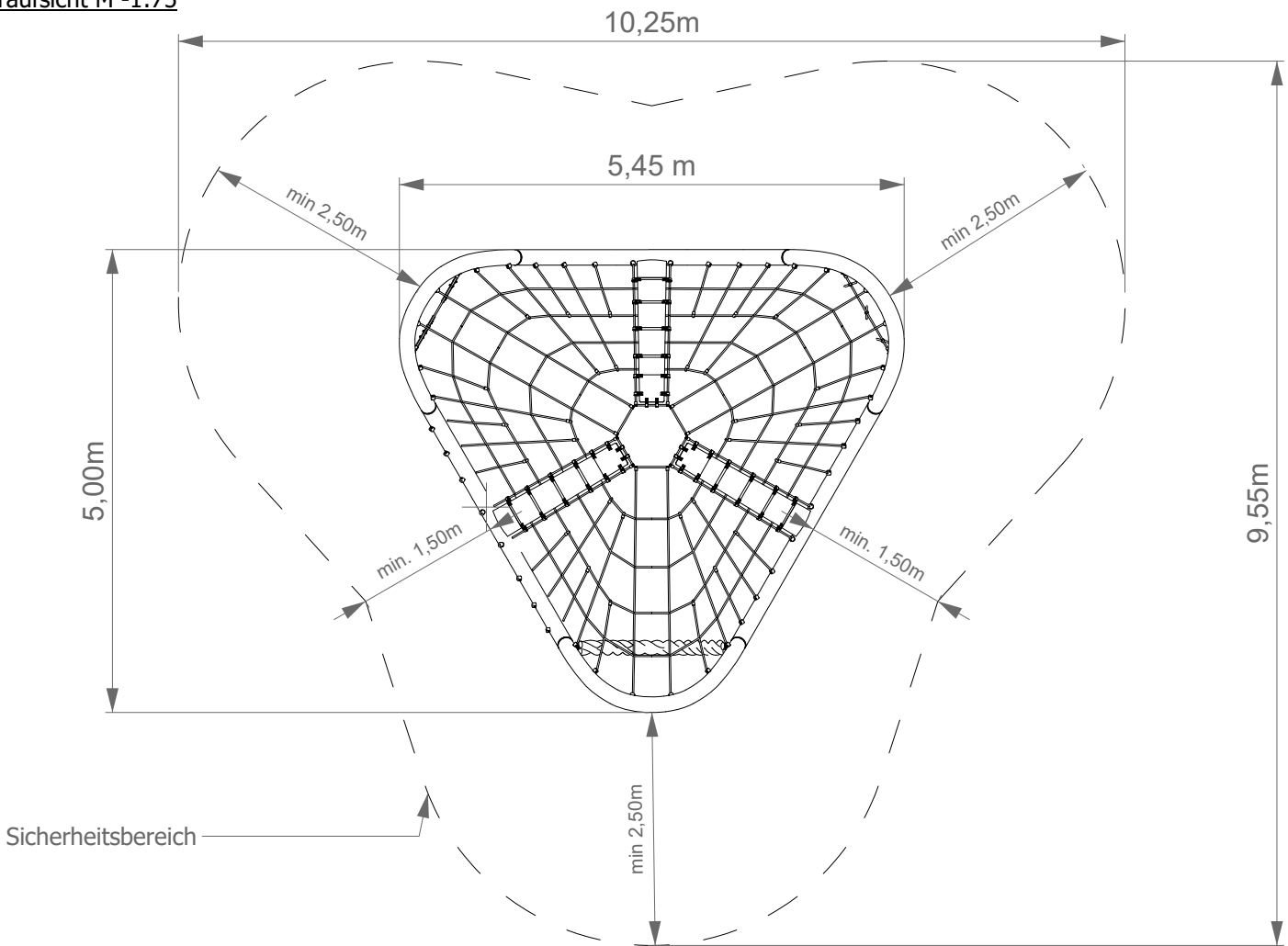
Draufsicht M -1:75
