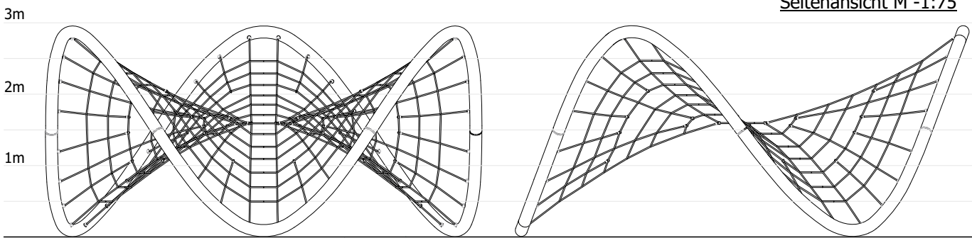
Seitenansicht M -1:75
