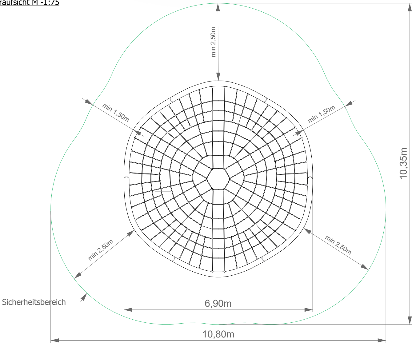
Draufsicht M -1:75
